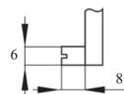
Dimenzije jezička ključa
