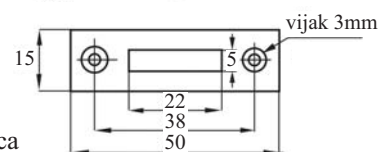
Priporna ploščica
